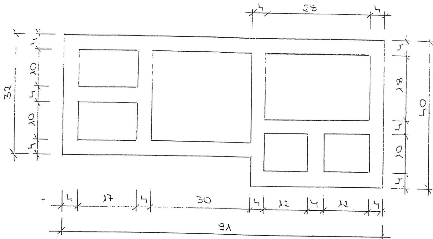
Rzut prefabrykatu elementu kominowego 6-cio kanałowego wentylacyjnego
